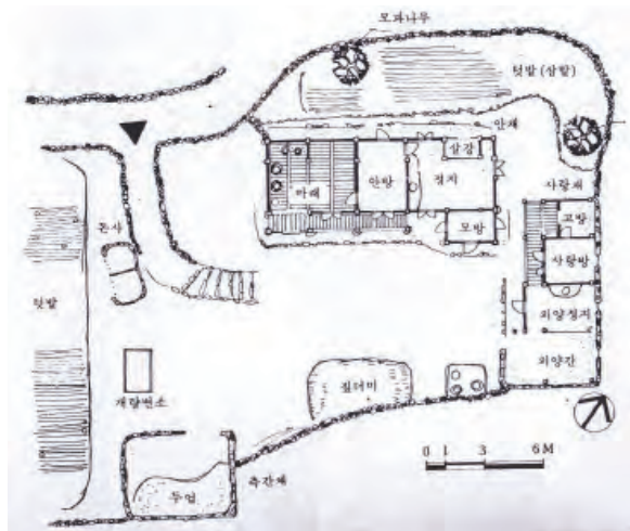
그림 4. 김성배 가옥 배치도
