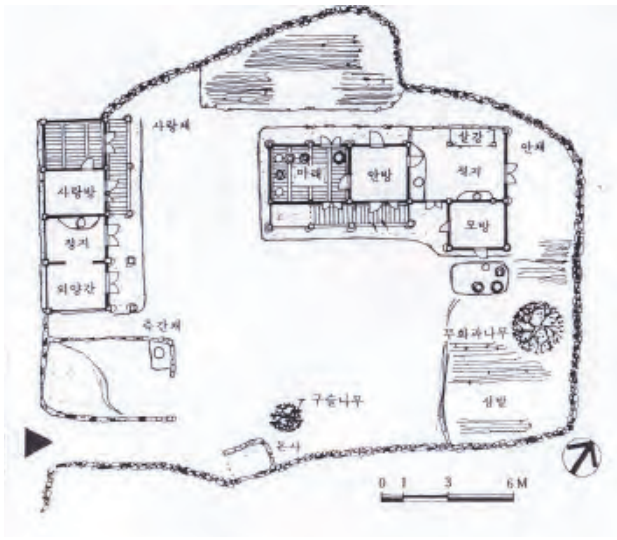
그림2. 제갈천일 가옥 배치도
