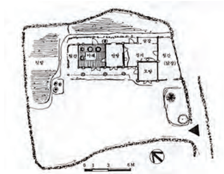
[도면2] 박문섭 가옥 배치도
